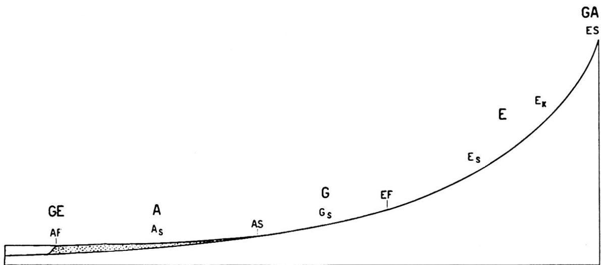
Fig. 25 Schema eines Normallängsprofils.
