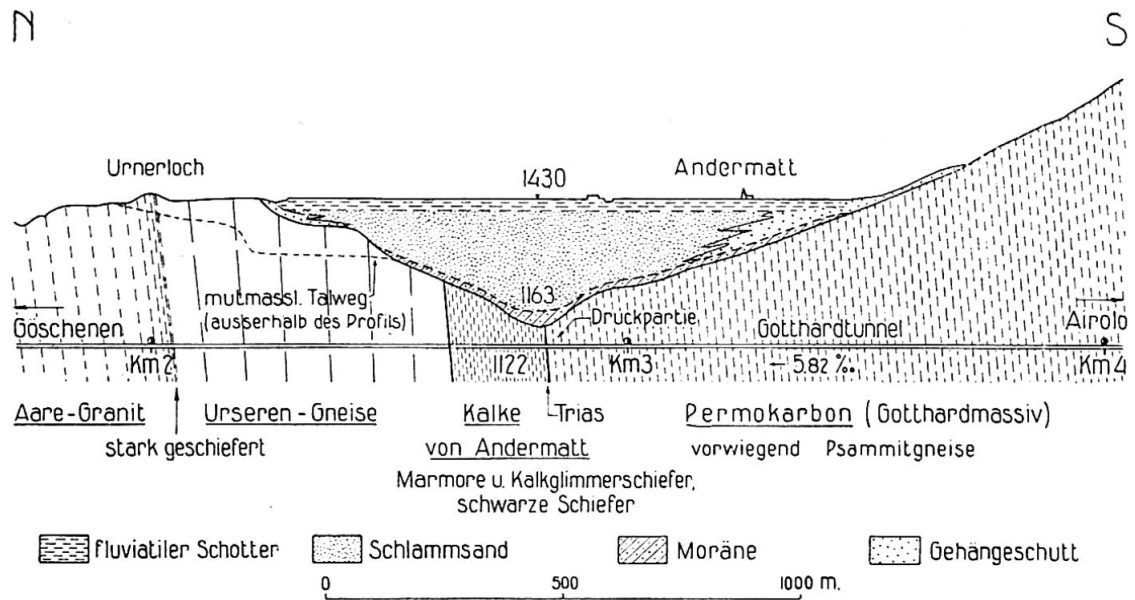
Fig. 37 Geologisches Profil 1:20 000 durch das Andermatt Becken in der Achse des Gotthardtunnels (nach E. Meyer-Peter, Th. Frey, A. Kreis und R. U. Winterhalter, 1945). Cliché aus E. NIGGLI 46 , mit freundlicher Bewilligung der Red. der Eclogae Geol. Helv.
