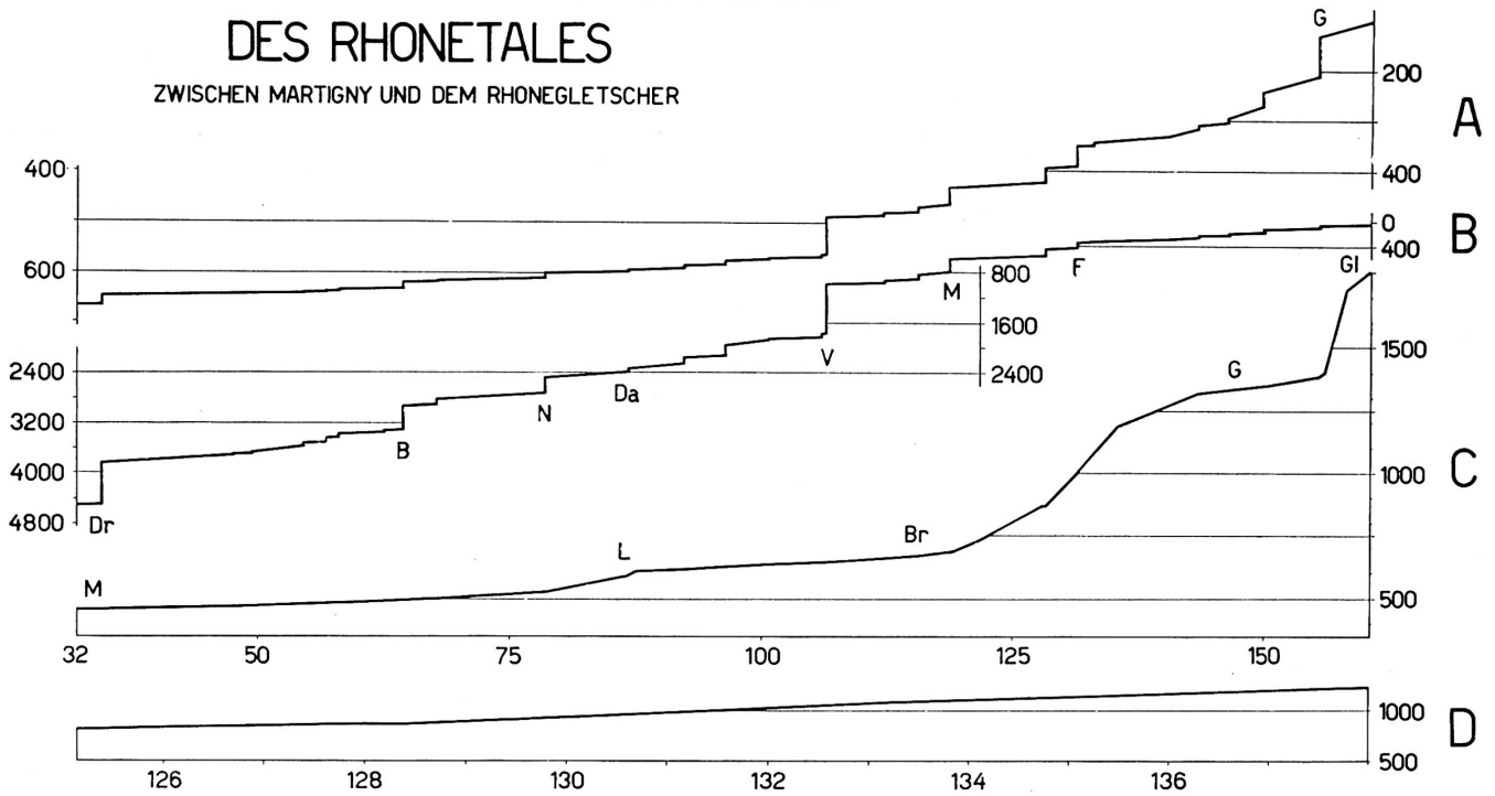
Fig. 36 Längenprofile und Summenkurven
