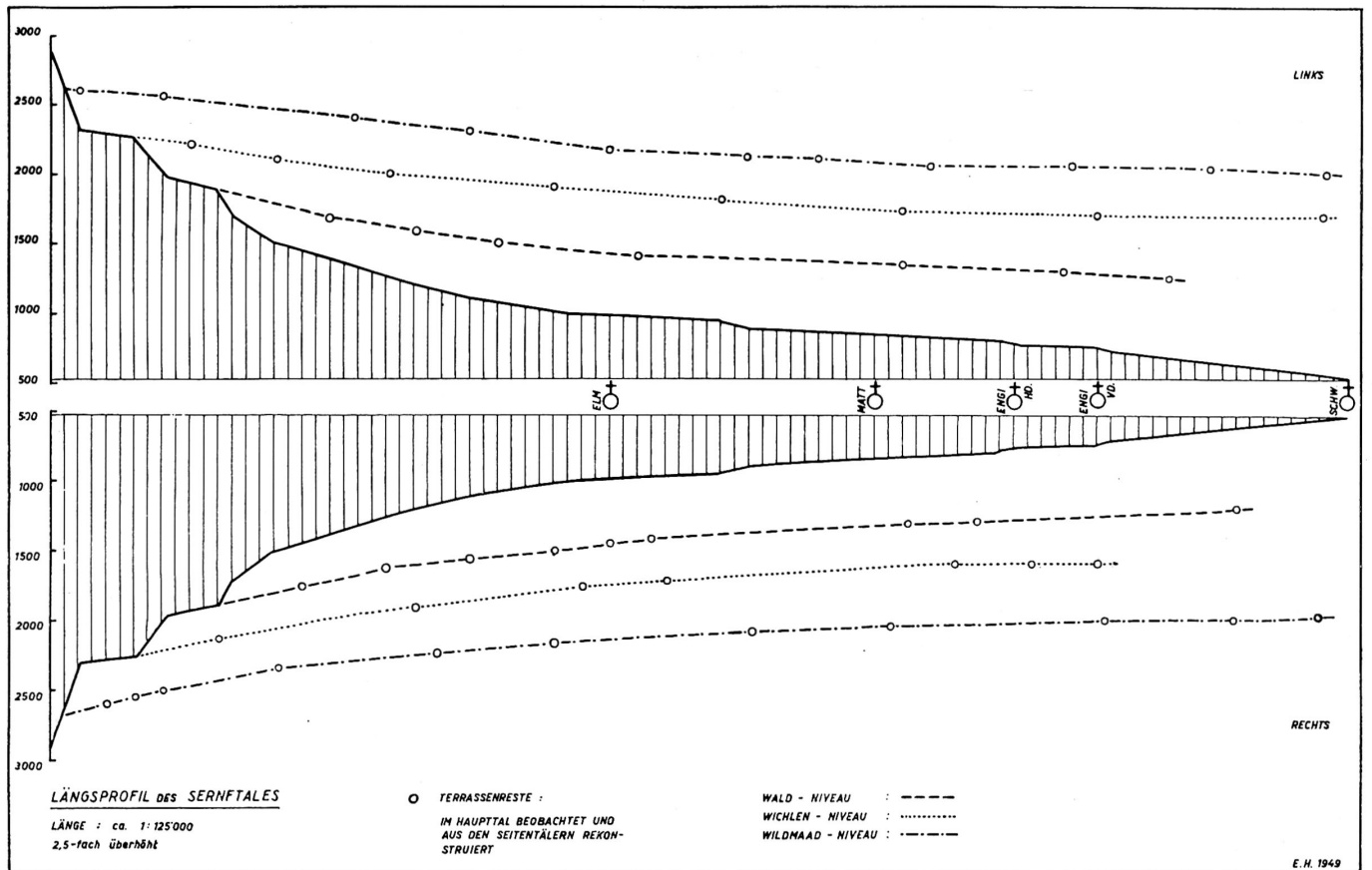
Fig. 42 Sehr schematische Rekonstruktion aus dem Serrfial. (Aus HEUBLING 27 , S. 136.)
