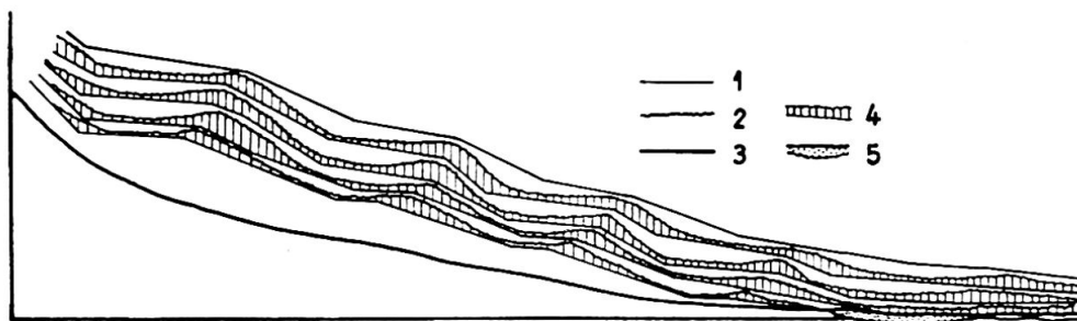
Fig. 38 Schema der Entwicklung des Längsprofils eines großen Alpentales nach DE MARTONNE 39 . 1. Fluviale präglaziale und interglaziale Profile. 2. Glaziale Profile. 3. « Profil d'équilibre ». 4. Inter- glaziale Tiefenerosion. 5. Interglaziale Aufschüttung.
