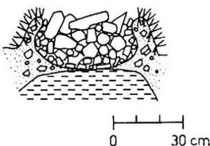
Fig. 2 Profil durch einen Steinring. Punktiert: Feinerde. Gestrichelt: Frostboden. V: Vegetation. Fig. 3 Profil durch den Wulst des Steinrings von Fig. 2. Fig. 4 Profil durch einen Streifen. Fig. 5 Profil durch einen Wulst eines deformierten Steinrings. Gefälle von links nach rechts. Fig. 6 Profil durch den Steinrahmen zweier benachbarter Polygone. Fig. 7 Profil durch den Steinrahmen eines schwach deformierten Polygons. Hangneigung 3° (Profil 5 liegt in der Fallinie, Profil 7 verläuft senkrecht zu ihr).
