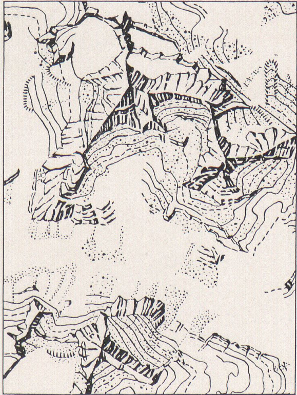
Abb. 2. Dasselbe Gebiet. Generalisierte Felszeichnung für eine Reliefkarte 1:100 000.
