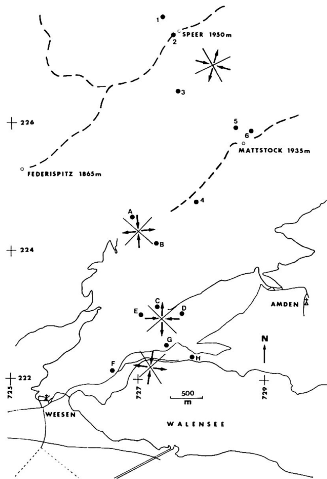
Abb. 6 Resultat der Klüftmessungen im Gebiet um Amden. Die Meßstellen sind mit 1–6 und A–H bezeichnet. Die bevorzugten Streichrichtungen der Klüfte in den Gruppen 1–6, AB, CDE und FGH sind durch gerade Linien bezeichnet, die daraus abgeleiteten Hauptspannungsrichtungen durch Pfeile.
