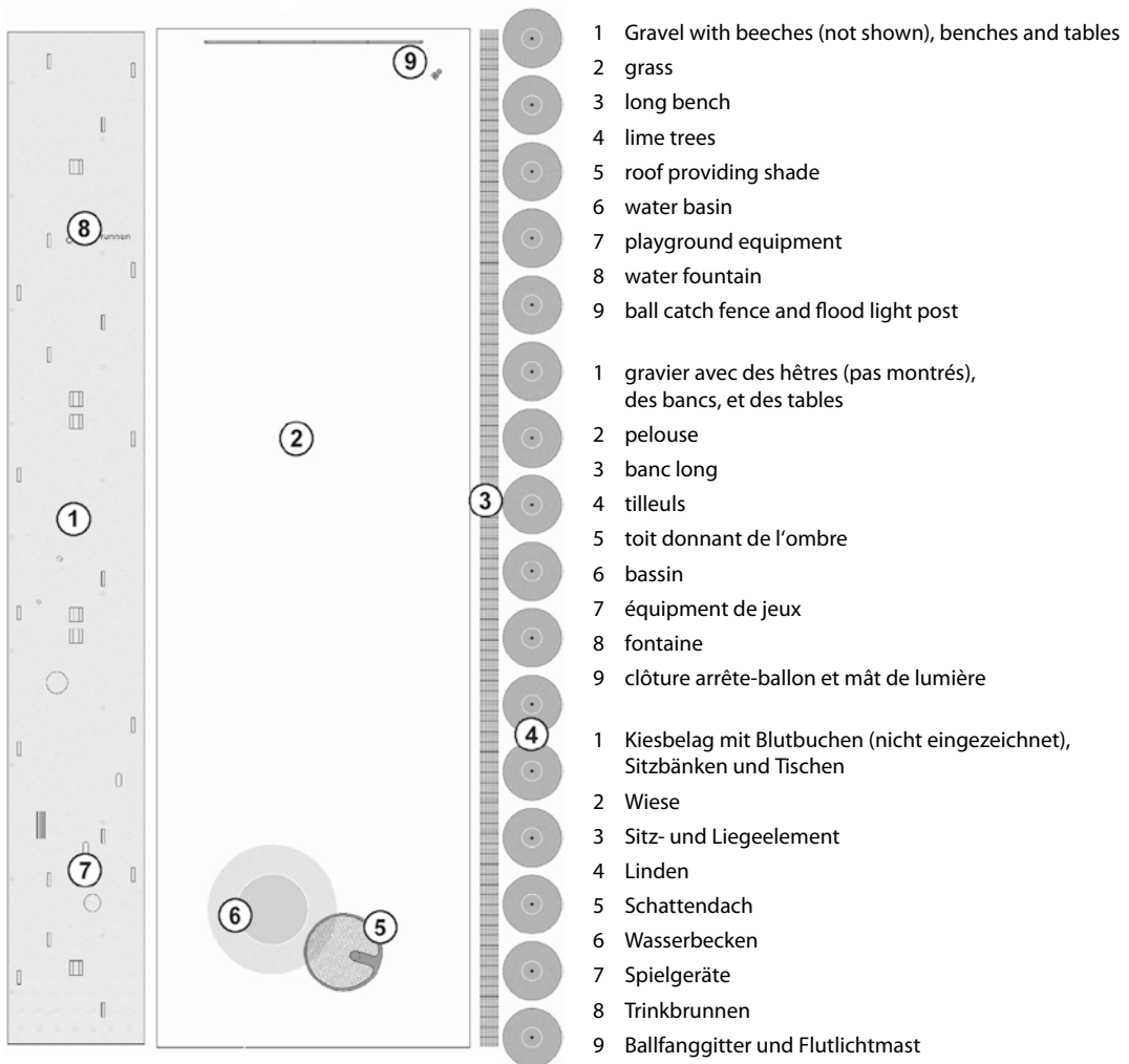
Fig. 1: Plan of Wahlenpark (Zurich, Switzerland)
